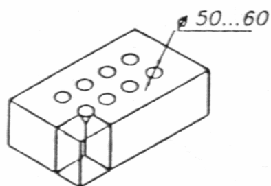
Рисунок А10 — Кирпич с 8 несквозными отверстиями (пустотность 11 %)
