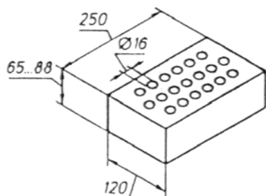
Рисунок А1 — Кирпич с 19 пустотами (пустотность 13 %)
