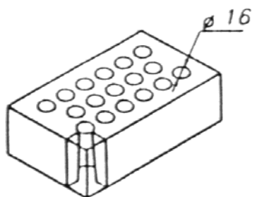
Рисунок А14 — Кирпич с 17 сквозными отверстиями (пустотность 12,7 %)
